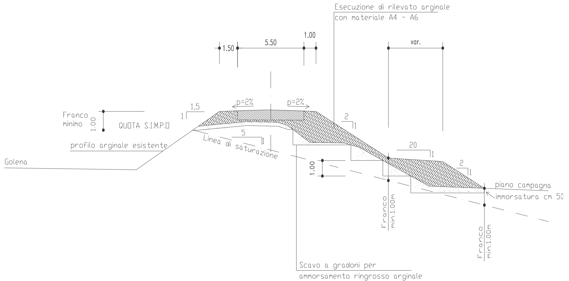
Esecuzione di rialzo e ringrosso arginale – medio Po
